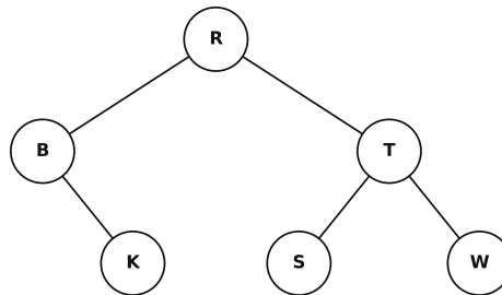
Figura 04 - Árvore Binária
