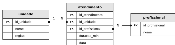
Figura 01 - Modelo Entidade-Relacionamento
